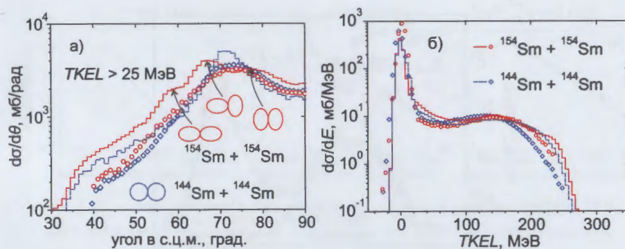
Рис. 2: (а) Угловые и (б) энергетические распределения продуктов реакции, полученные в реакциях ^{144}\text{Sm} + ^{144}\text{Sm} и ^{154}\text{Sm} + ^{154}\text{Sm} при энергиях E_{c.m.} = 500 и 485 МэВ соответственно. Гистограммами обозначены результаты расчётов, а символы показывают экспериментальные данные [19]. Пунктирная гистограмма и ромбы соответствуют реакции ^{144}\text{Sm} + ^{144}\text{Sm} , сплошная гистограмма и кружки — реакции ^{154}\text{Sm} + ^{154}\text{Sm} .
