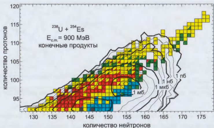
Рис. 7: Сечения образования конечных продуктов в реакции ^{238}\text{U} + ^{254}\text{Es} при E_{\text{с.м.}} = 900 МэВ, изображённые поверх карты известных нуклидов. Контурные линии показывают величину сечения в логарифмическом масштабе с шагом в один порядок.
