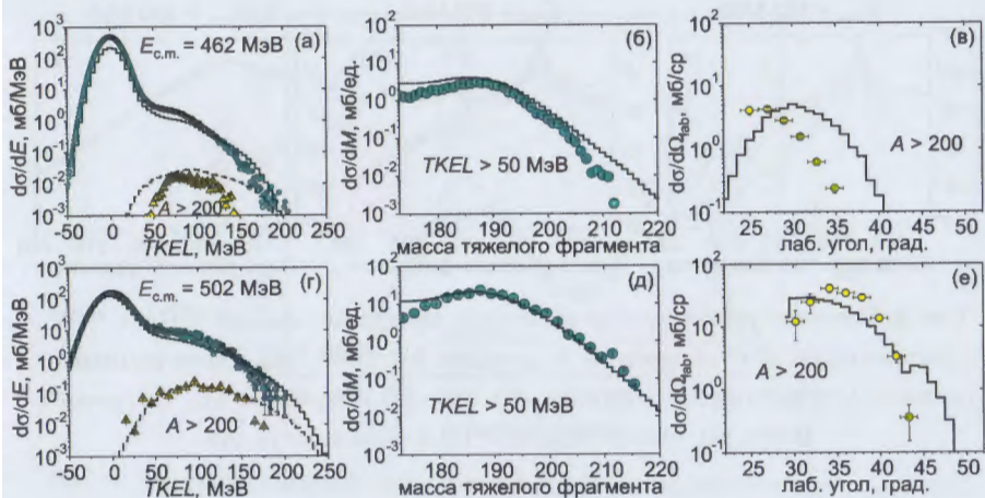
Рис. 5: Энергетические, массовые и угловые распределения первичных продуктов, полученных в реакции ^{160}\text{Gd} + ^{186}\text{W} при двух энергиях E_{c.m.} = 462 и 502 МэВ. Символами обозначены экспериментальные данные [12], жирные гистограммы показывают результаты расчётов, усреднённые по взаимным ориентациям ядер снаряда и мишени. Треугольниками и штриховыми гистограммами обозначены энергетические распределения, соответствующие мишенеподобным фрагментам с A > 200 . В расчётах учитывалось экспериментальное разрешение (FWHM) 12 МэВ по энергии и 3 единицы по массе.
