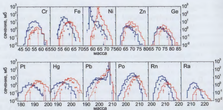
Рис. 1: Изотопные распределения конечных снарядо- и мишенеподобных фрагментов, образующихся в двух реакциях: ^{58}\text{Ni} + ^{208}\text{Pb} при энергии E_{c.m.} = 270 МэВ (сплошные ромбы и толстые гистограммы) и ^{64}\text{Ni} + ^{208}\text{Pb} при энергии E_{c.m.} = 268 МэВ (открытые треугольники и тонкие гистограммы).
